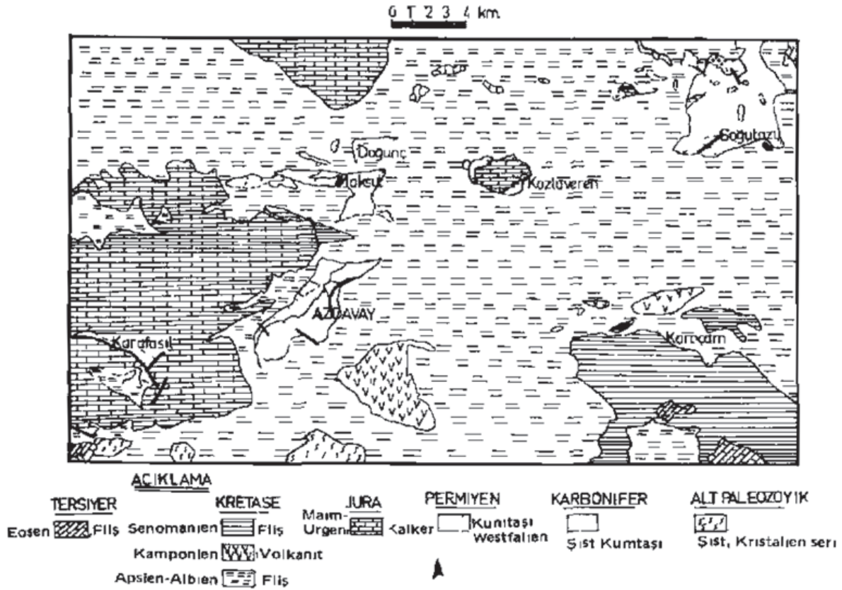
Şekil 1: Azdavay-Söğütözü Jeolojisi ve Kömür Varlığı
